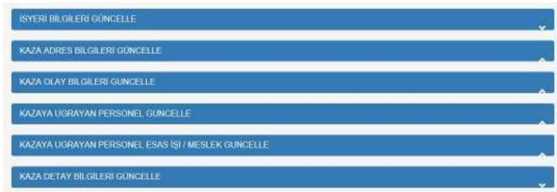
Şekil 27- Güncelleme ekranı
