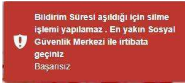
Şekil 26-Silme uyarı ekranı
